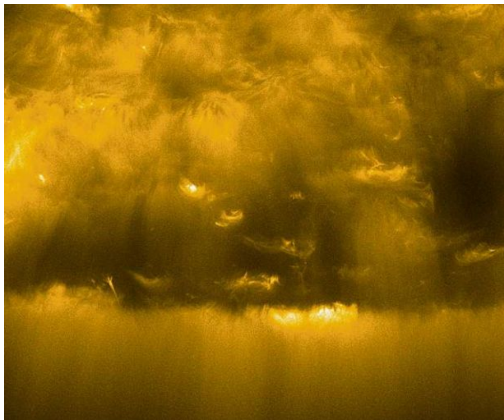
Solarer Südpol mit neuentdeckten, hochauflösenden Plasmastrukturen. Bild: ESA/Solar Orbiter/EUI Team
